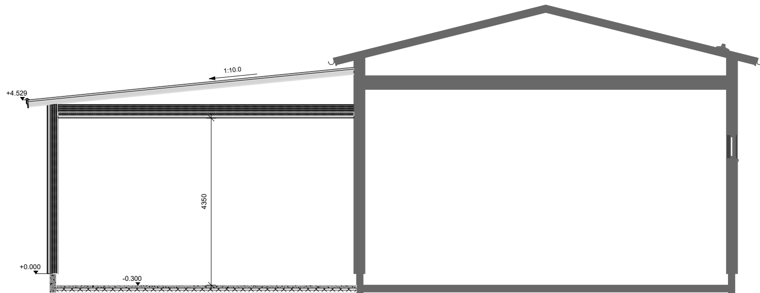
LEIKKAUS A-A
