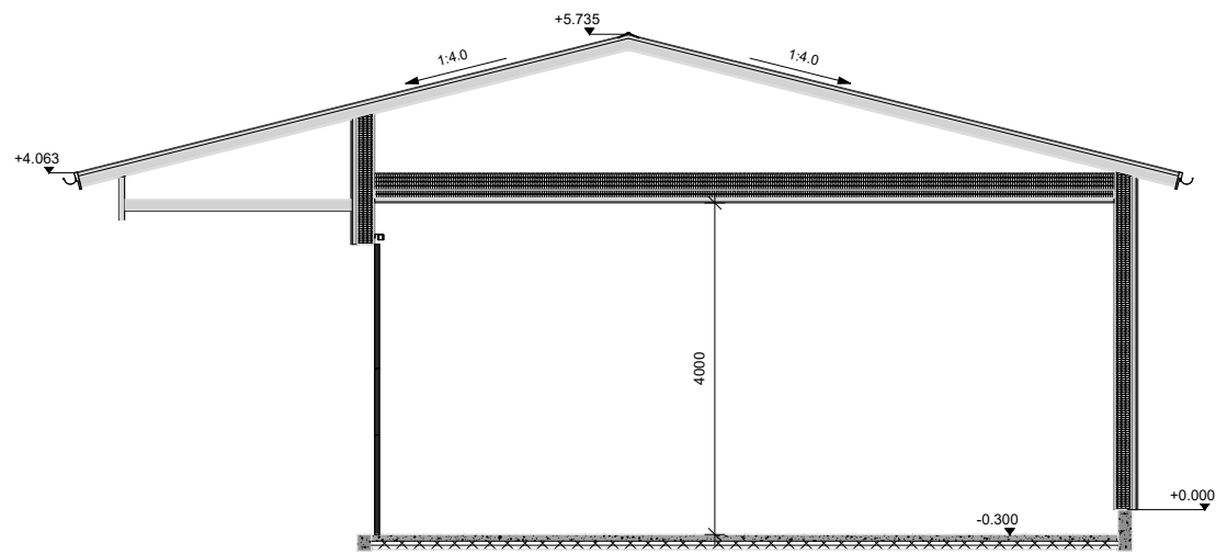
LEIKKAUS A-A
