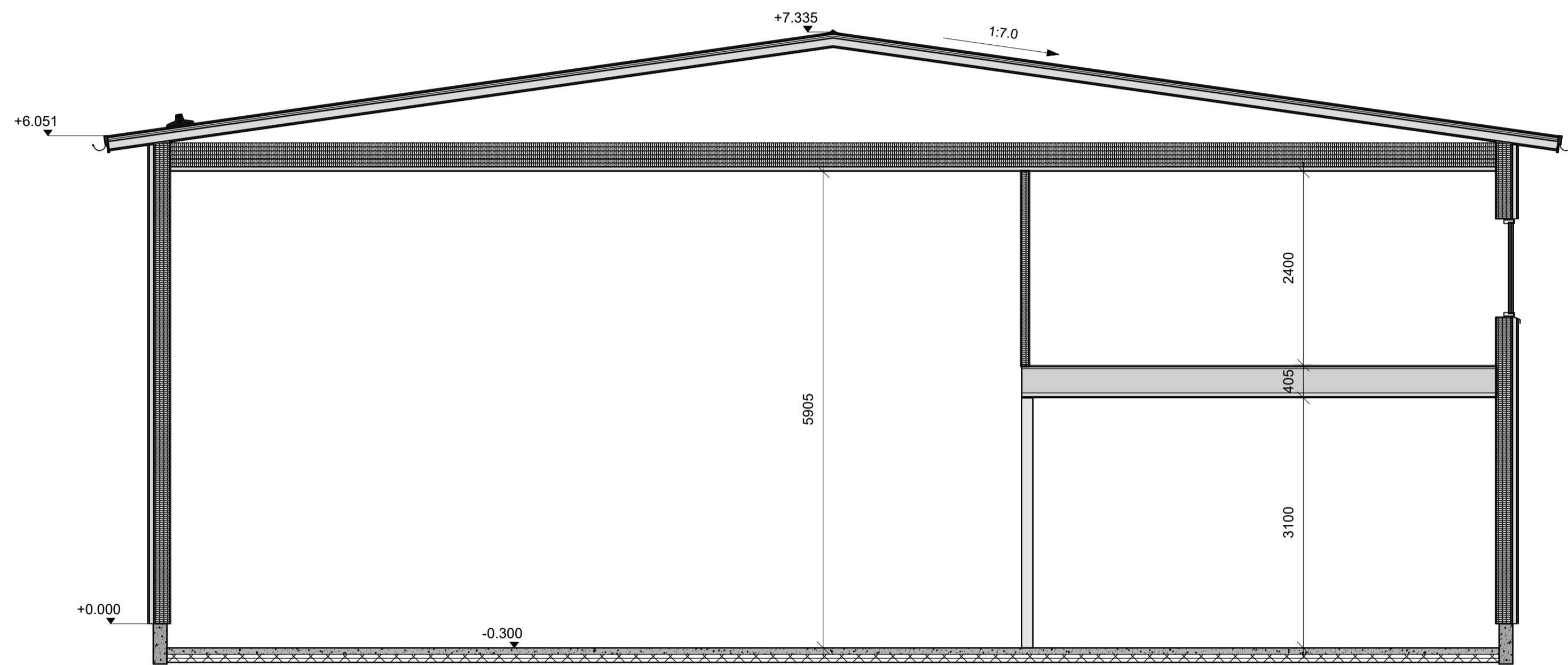
LEIKKAUS A-A
