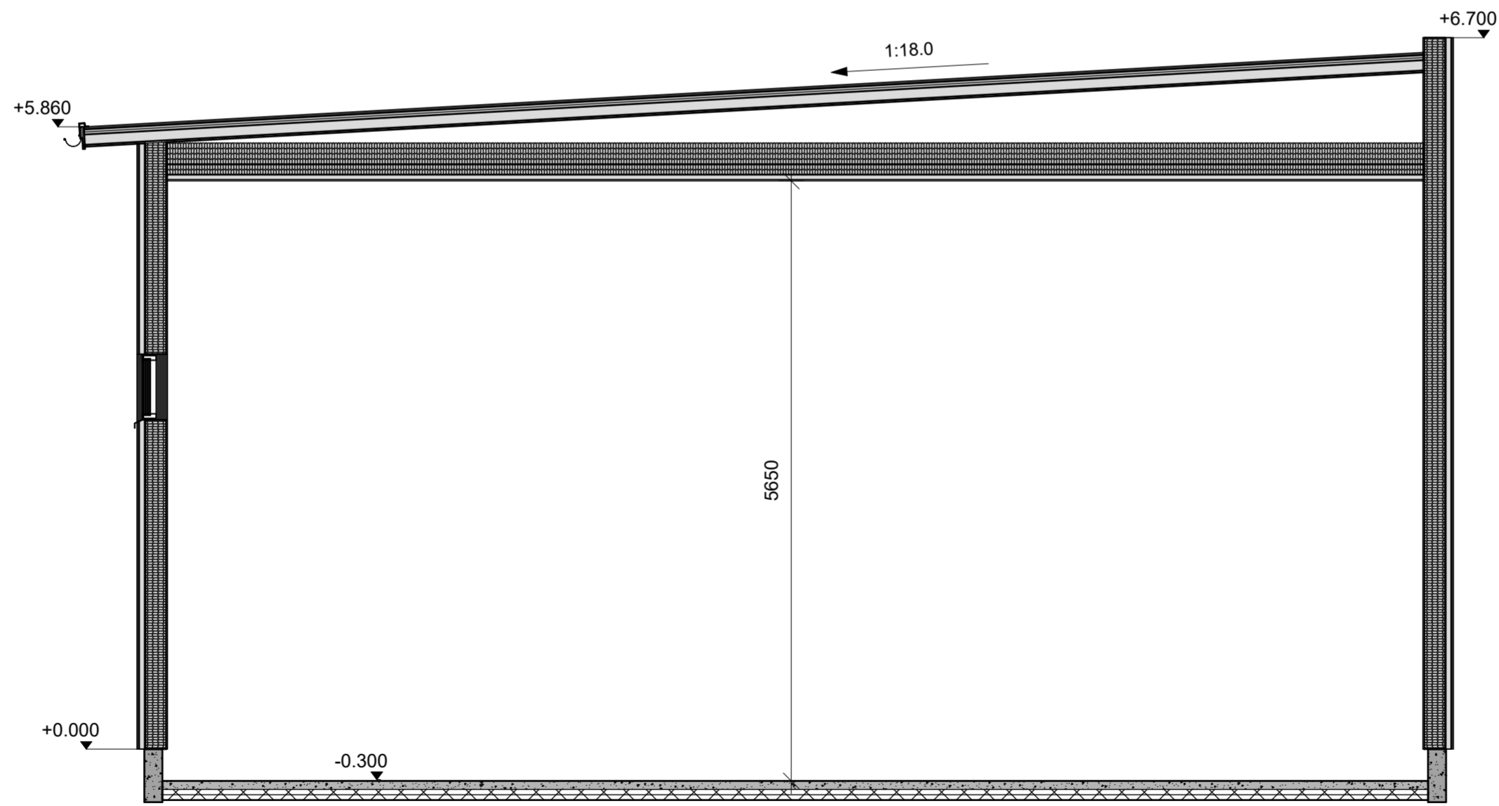
LEIKKAUS A-B
