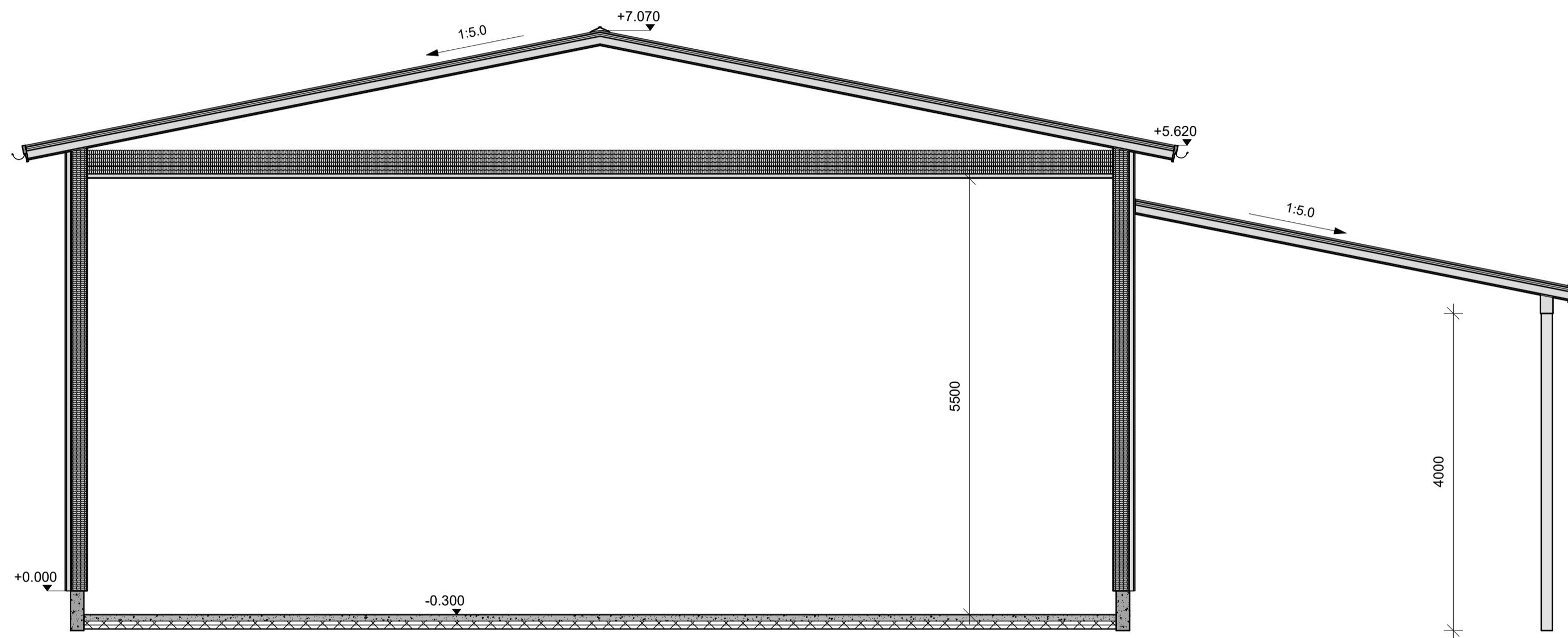
LEIKKAUS A-A
