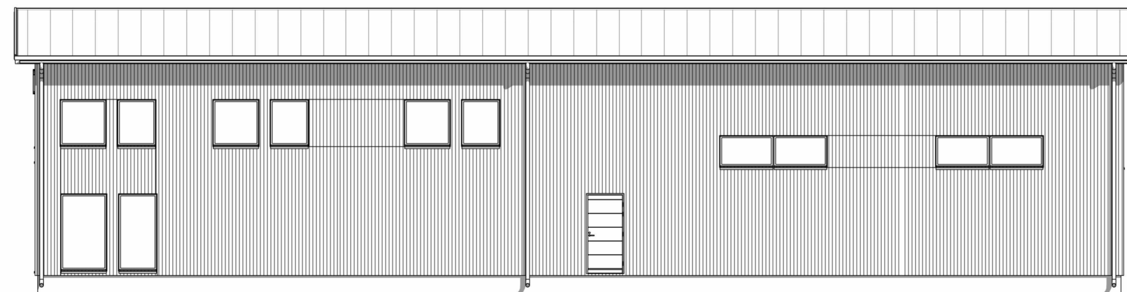
Julkisivu 3
