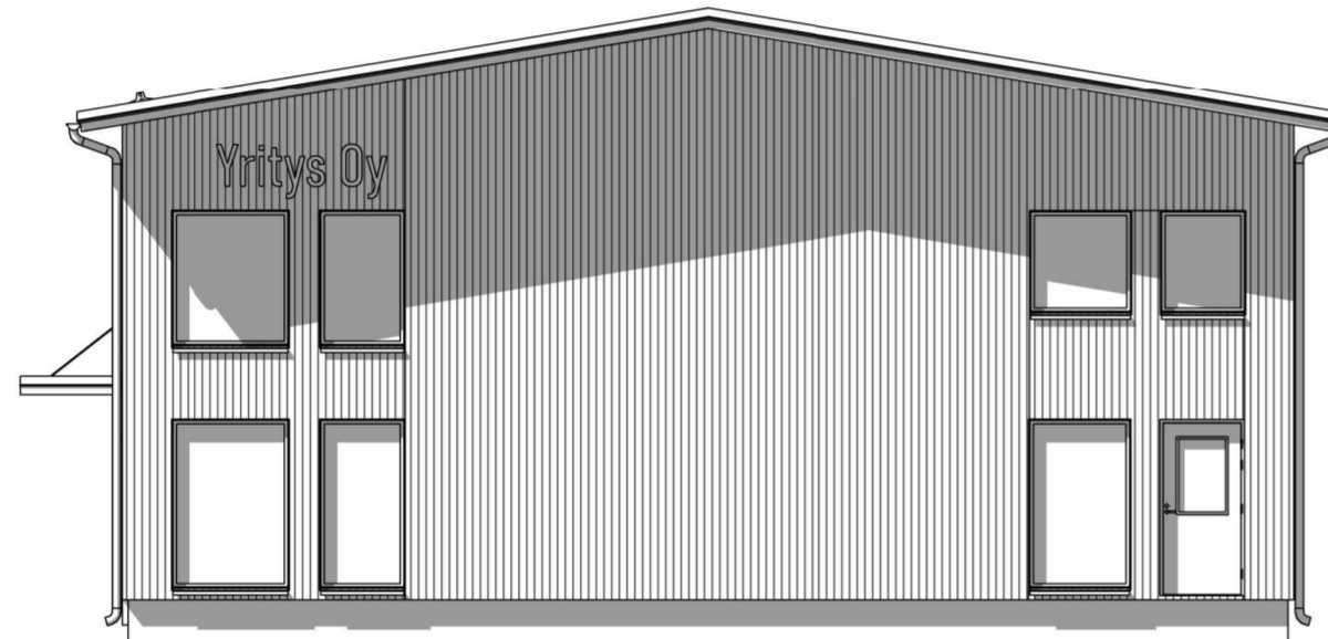
Julkisivu 2
