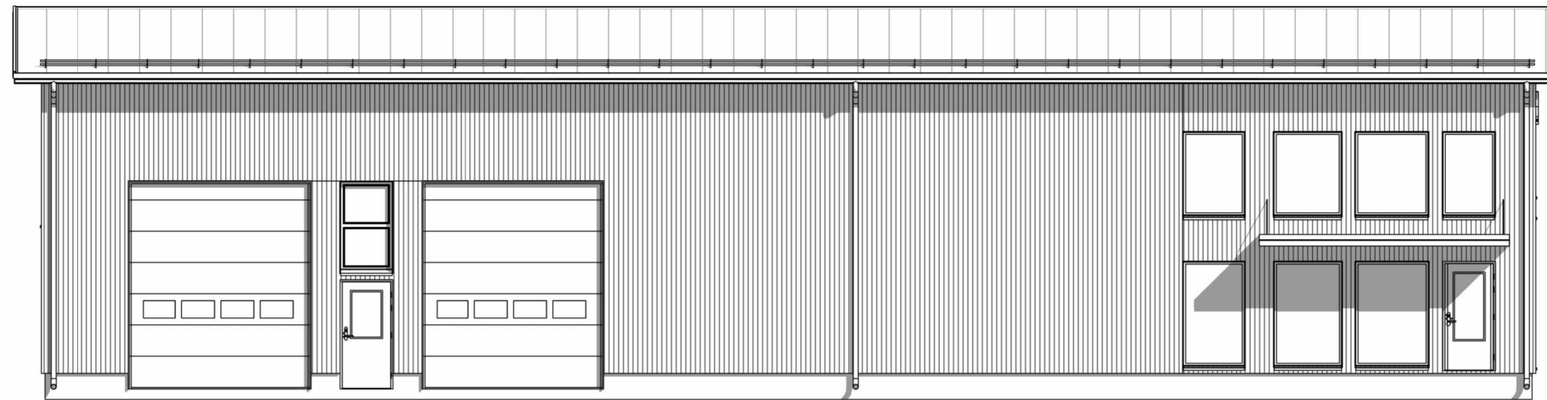
Julkisivu 1
