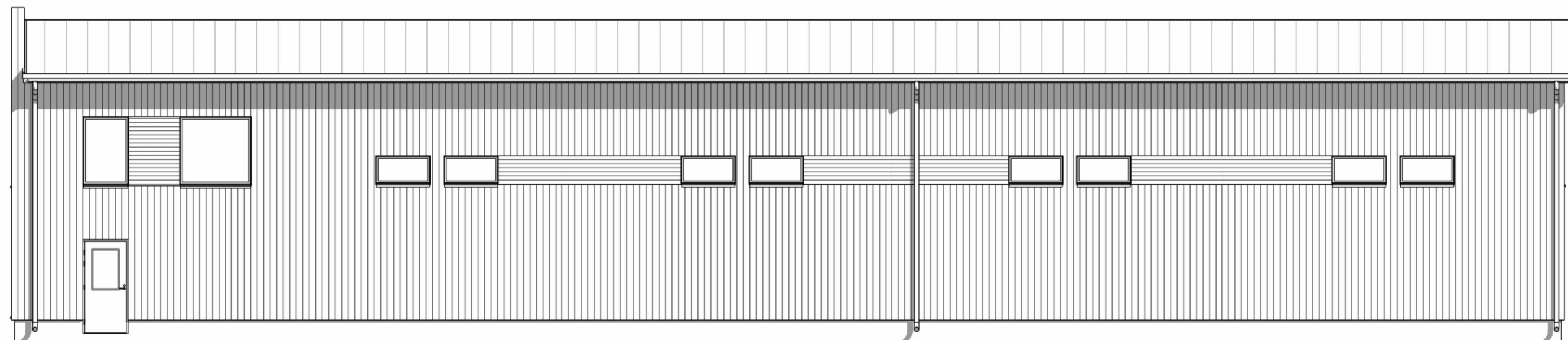
Julkisivu 3
