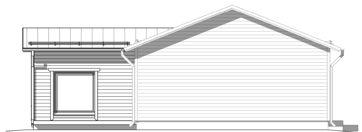
Julkisivu 1
