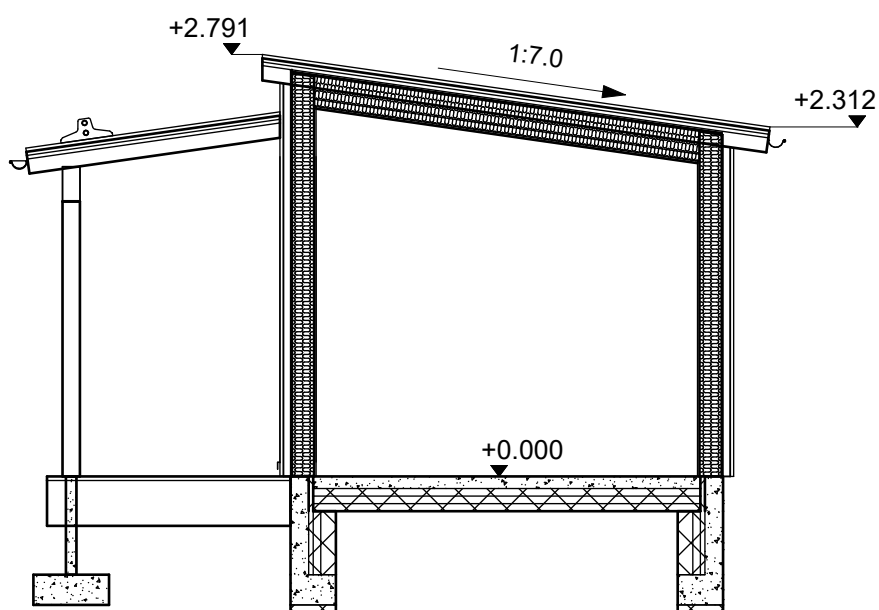
LEIKKAUS A-A
