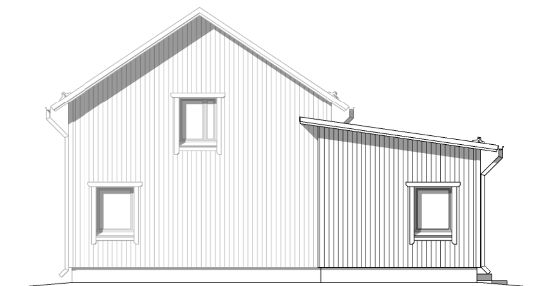
Julkisivu 4
