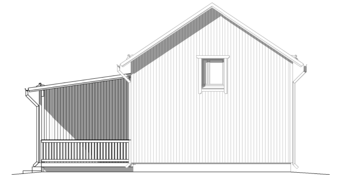
Julkisivu 2
