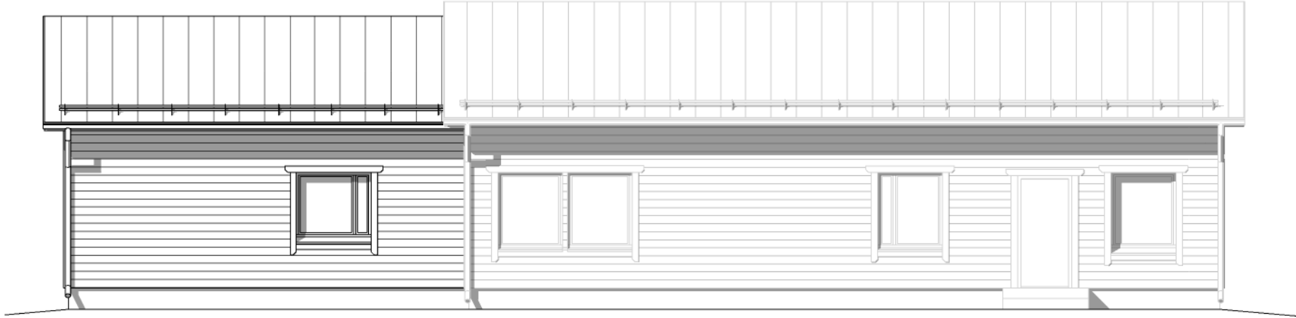
Julkisivu 3
