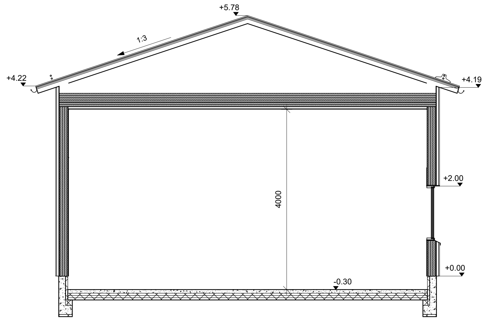
LEIKKAUS A-A
