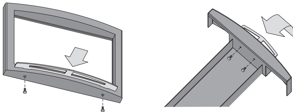
Kuva 16. Kahvojen kiinnittäminen
