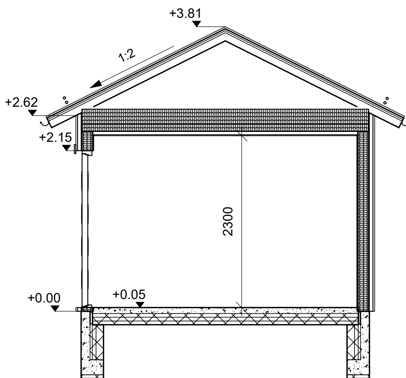
LEIKKAUS A-A
