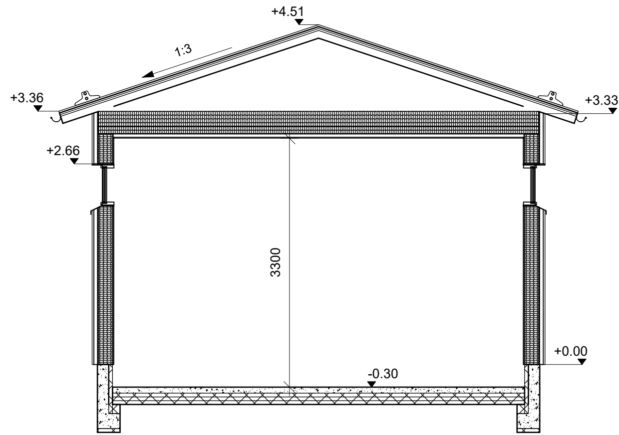
LEIKKAUS A-A
