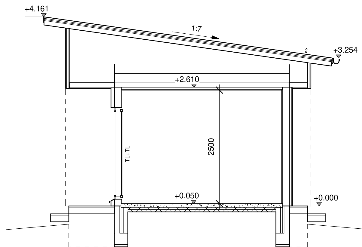
LEIKKAUS B-B
