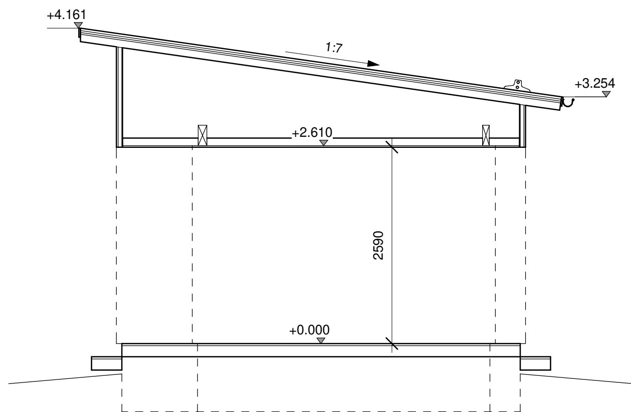
LEIKKAUS A-A
