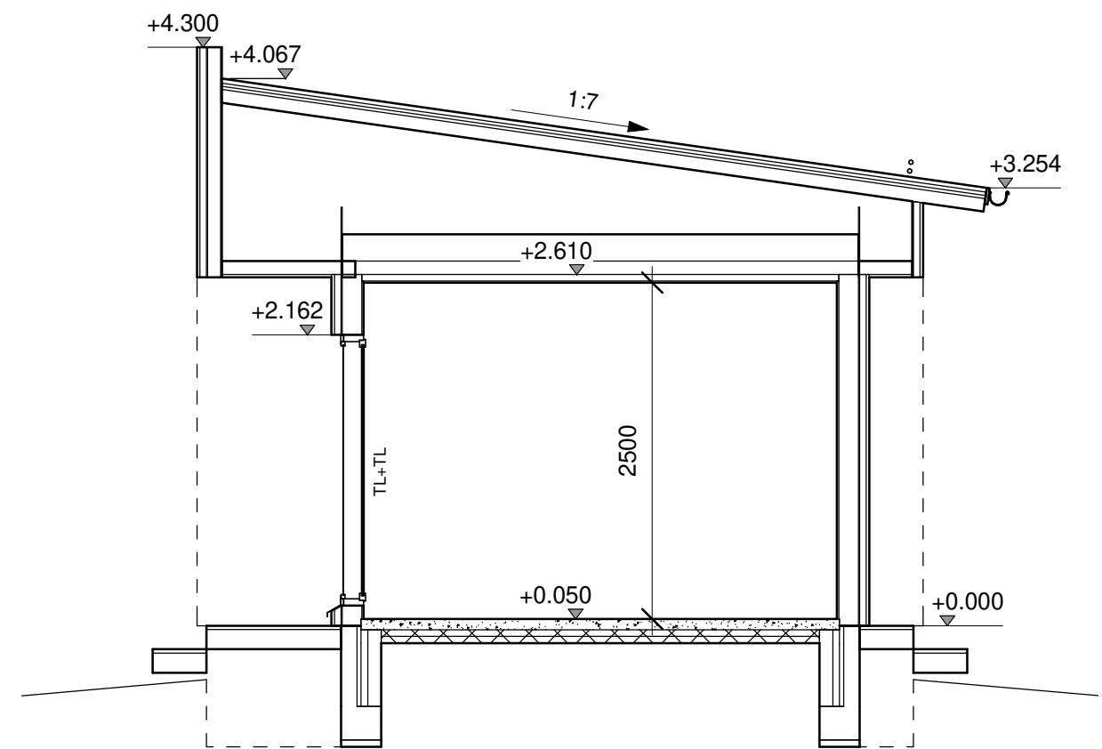
LEIKKAUS B-B
