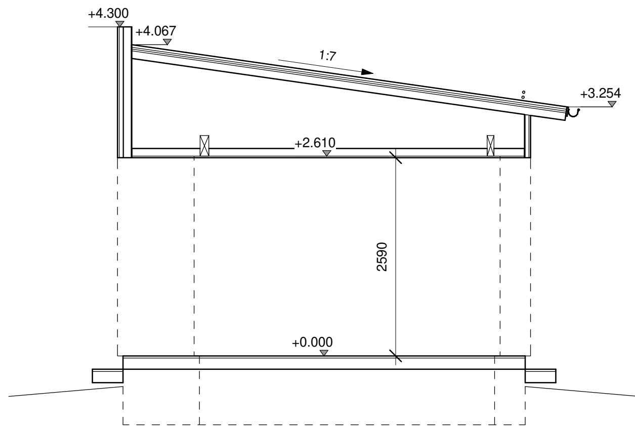
LEIKKAUS A-A
