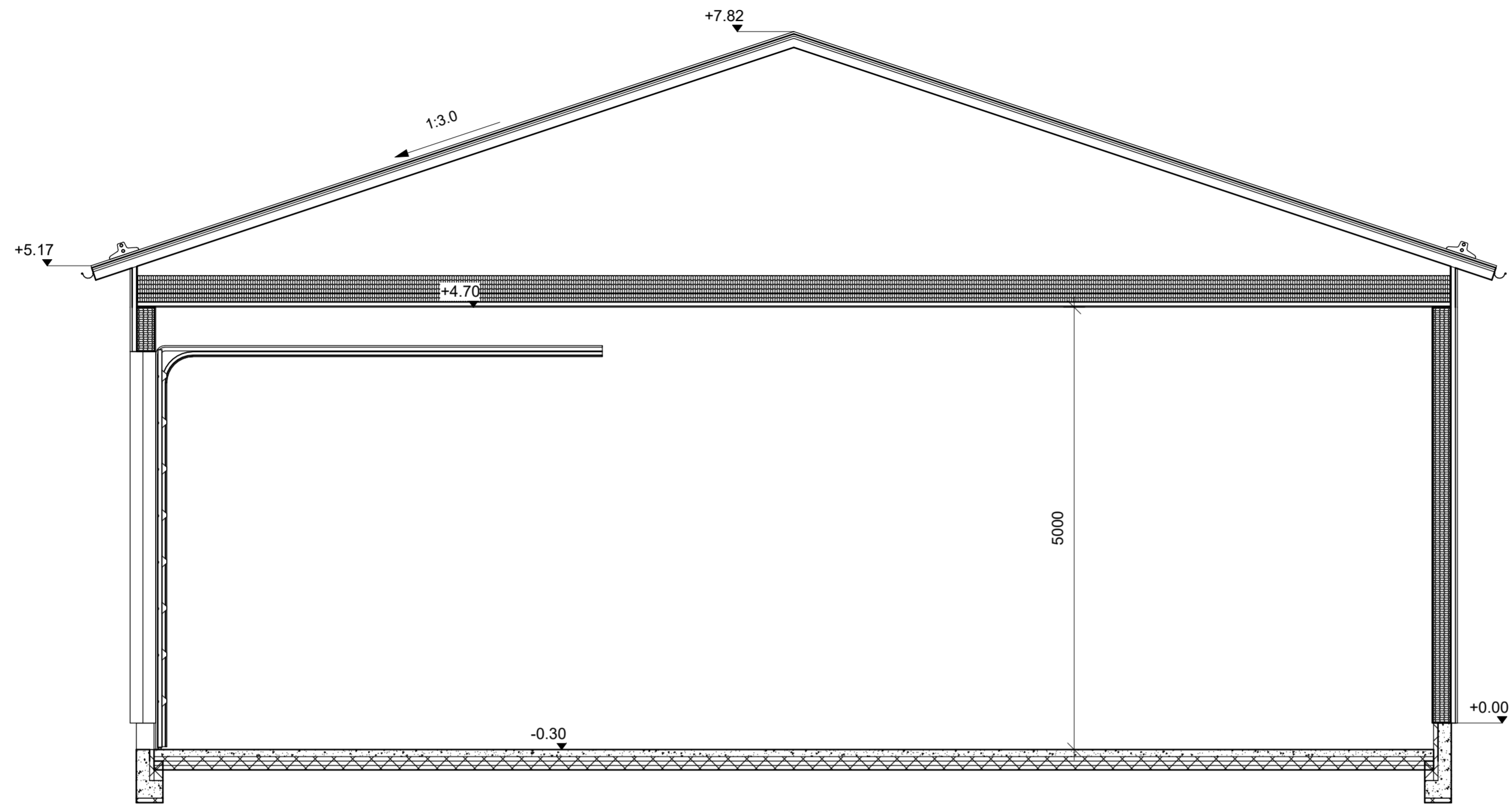
LEIKKAUS A-A
