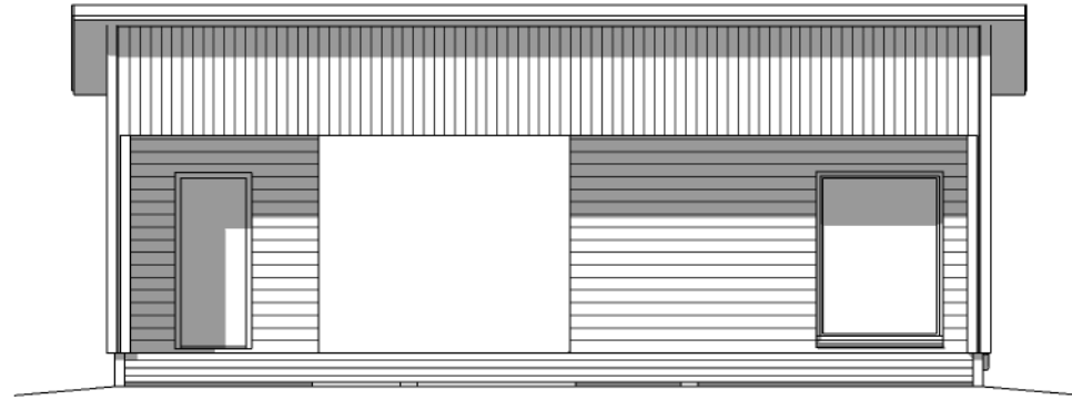
Julkisivu 1
