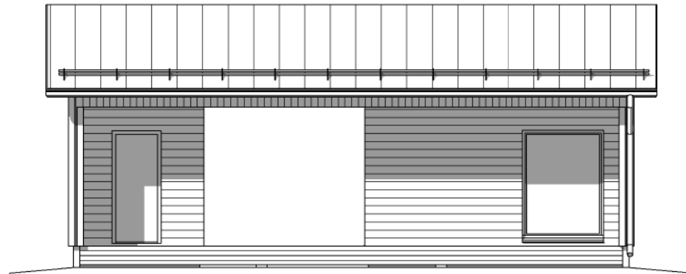
Julkisivu 1
