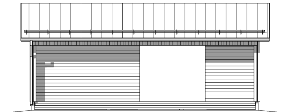
Julkisivu 3
