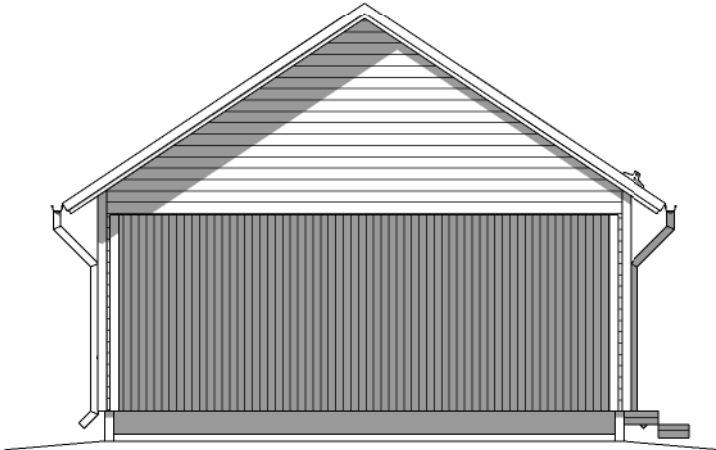
Julkisivu 2
