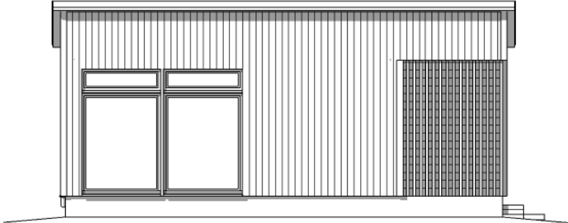
Julkisivu 1
