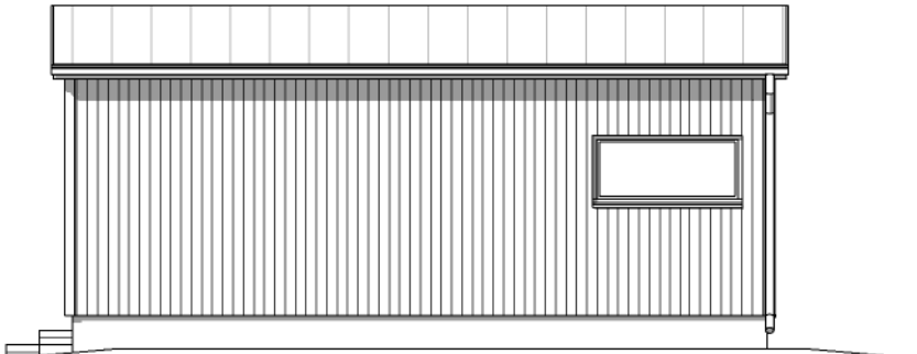
Julkisivu 3
