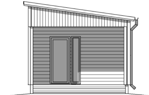
Julkisivu 4
