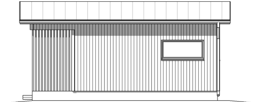
Julkisivu 3
