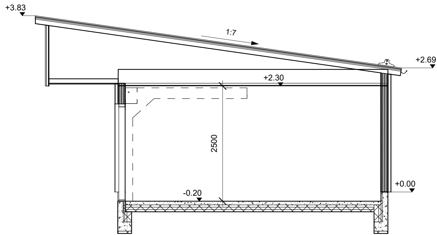
LEIKKAUS A-A
