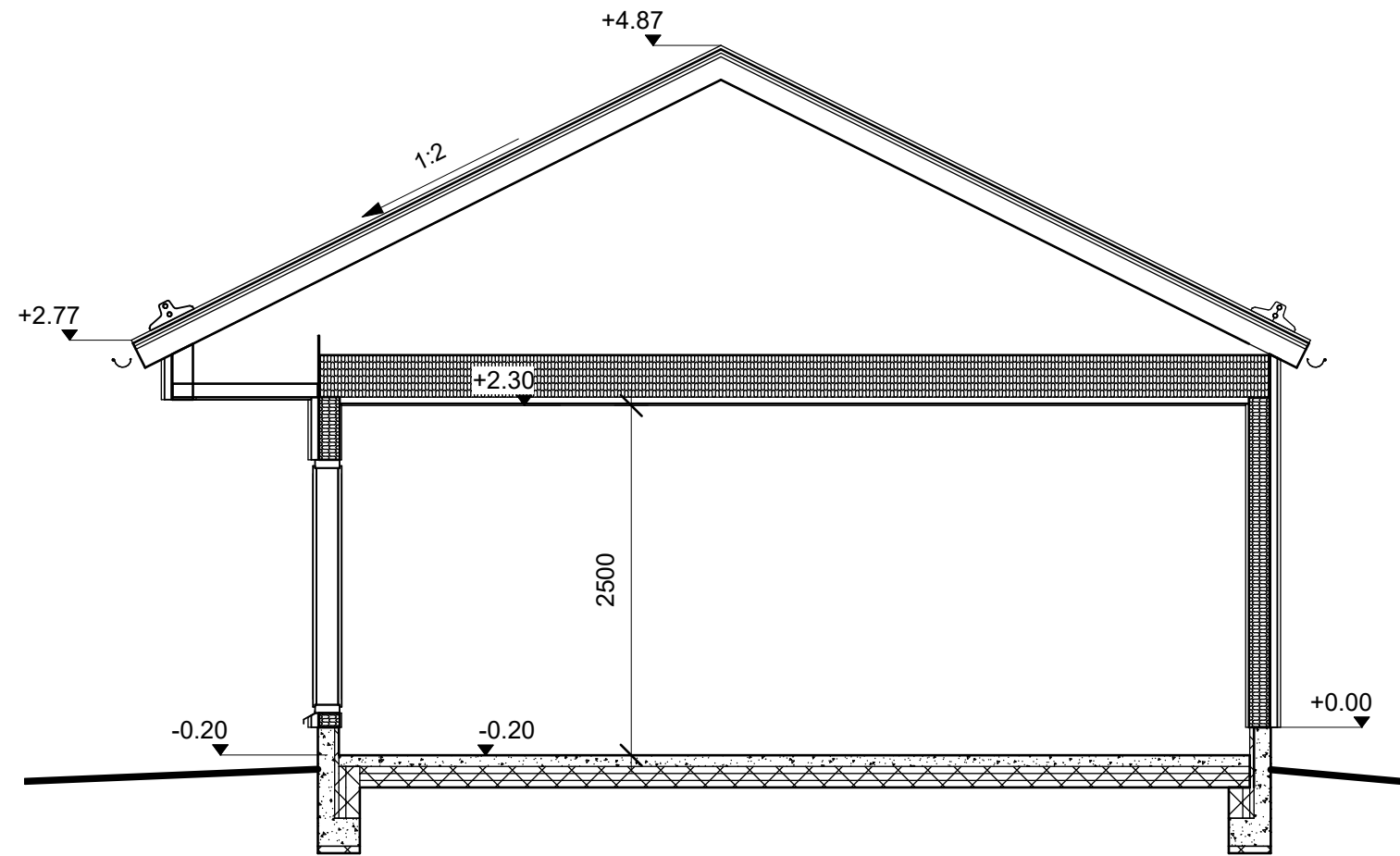
LEIKKAUS A-A
