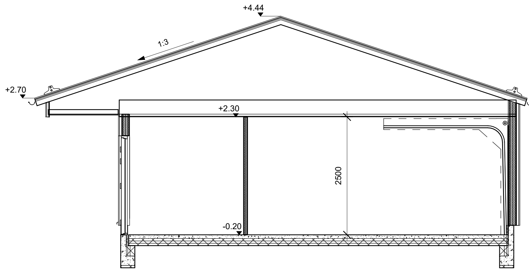
LEIKKAUS A-A
