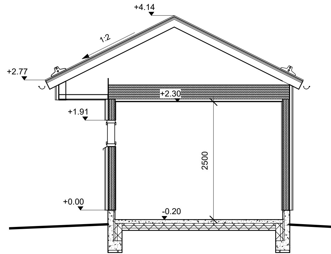
LEIKKAUS A-A
