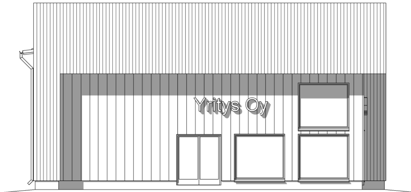
Julkisivu 2
