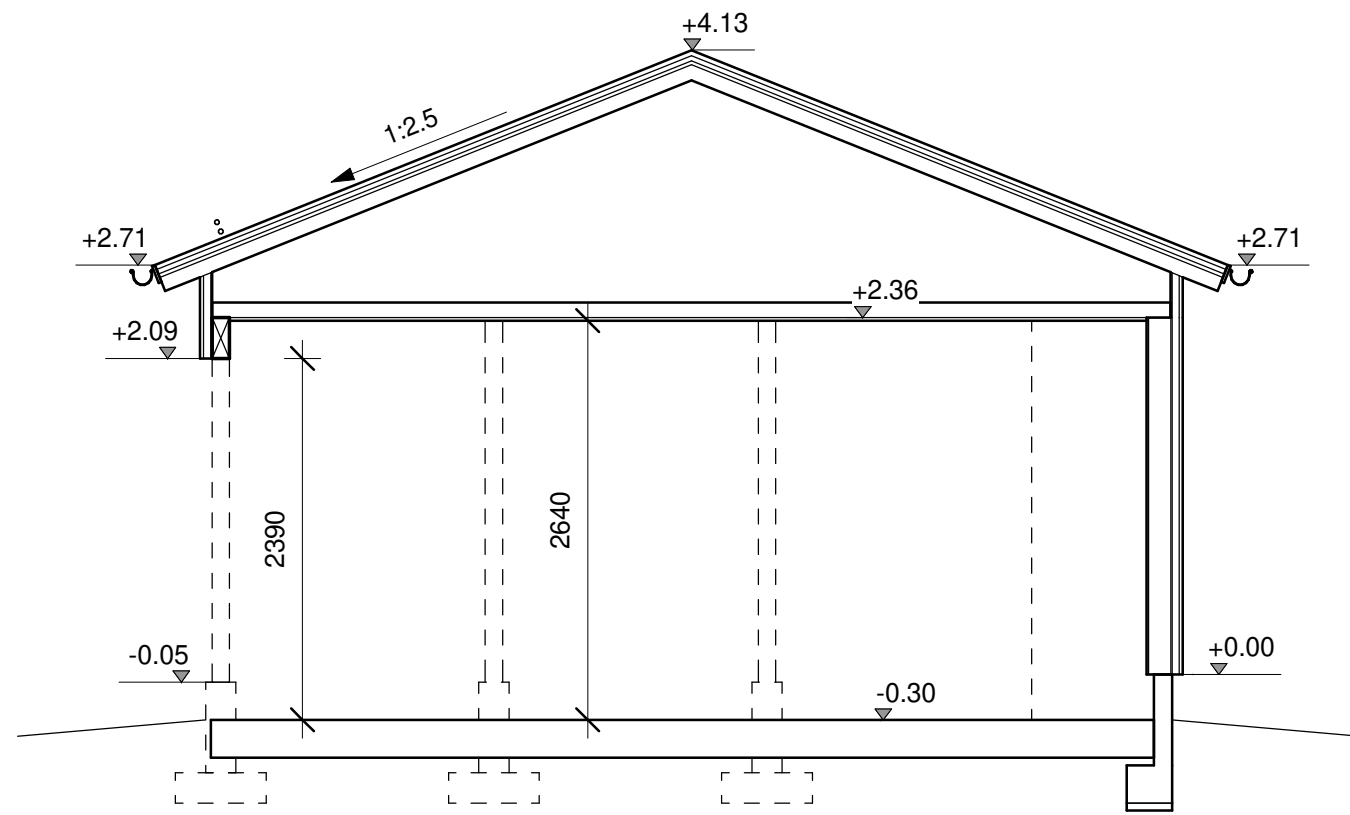
LEIKKAUS A-A
