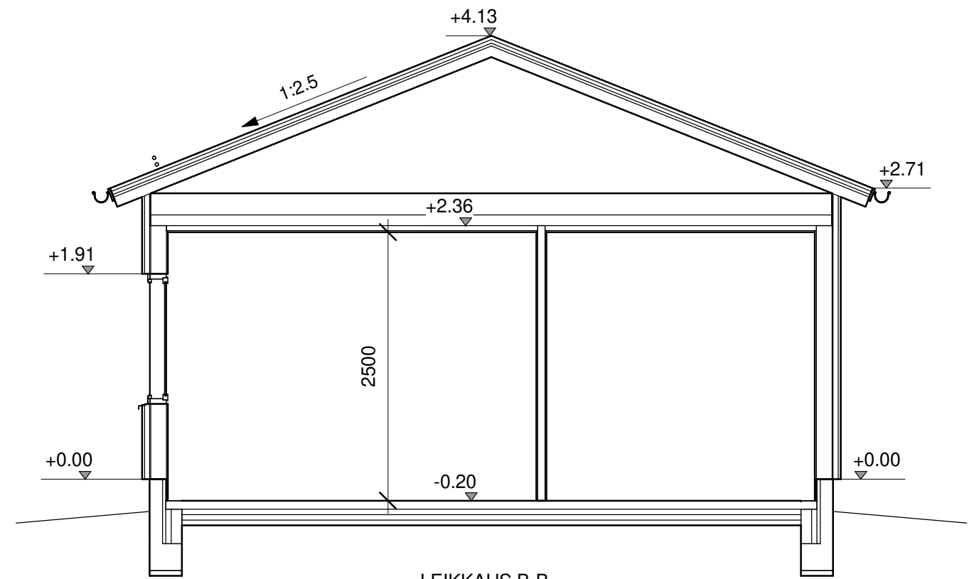
LEIKKAUS B-B
