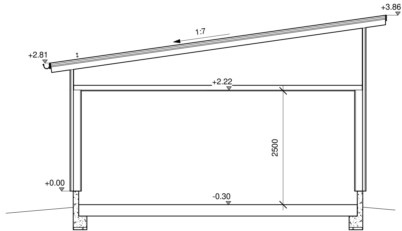
LEIKKAUS A-A
