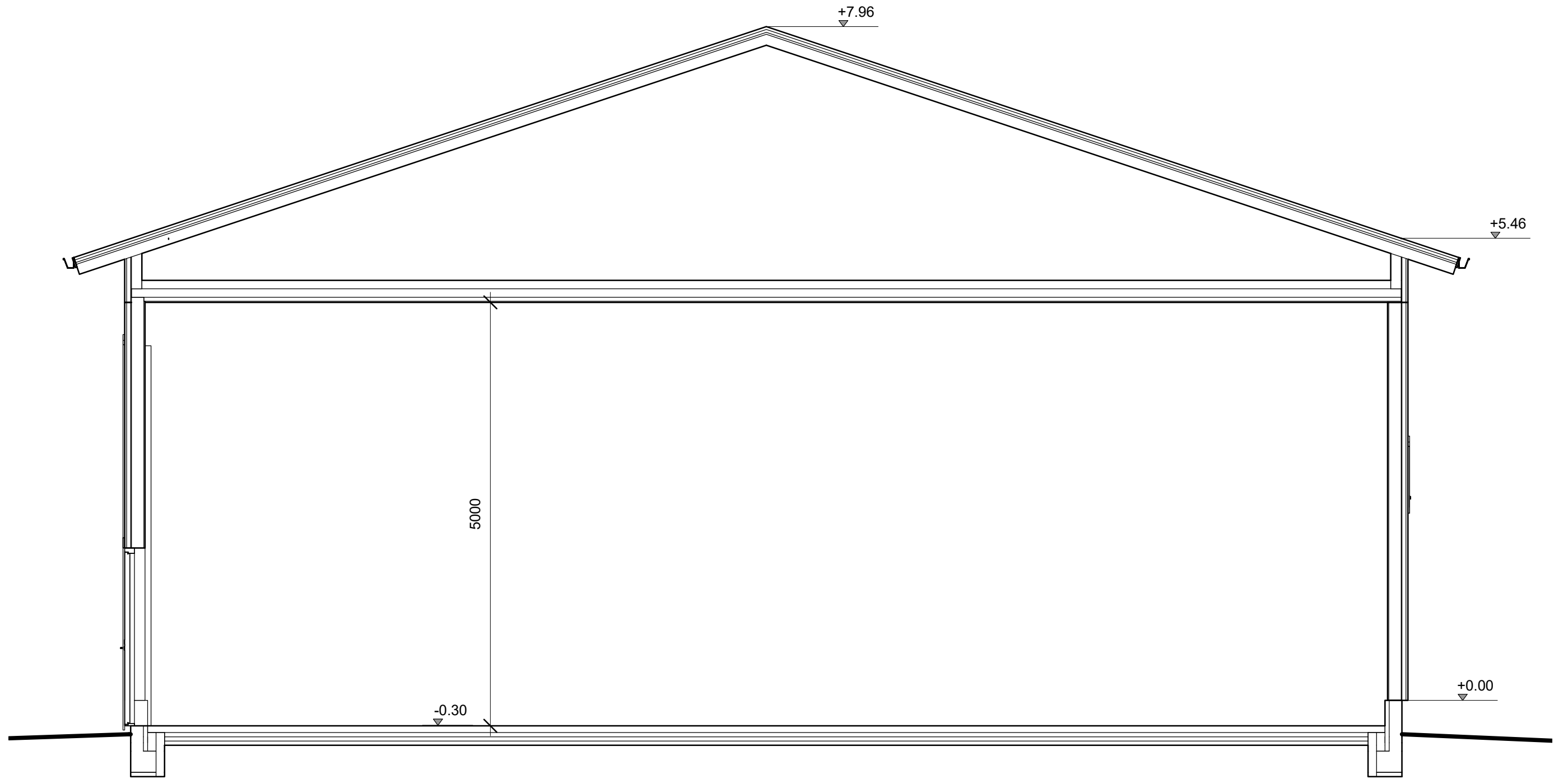
LEIKKAUS A-A
