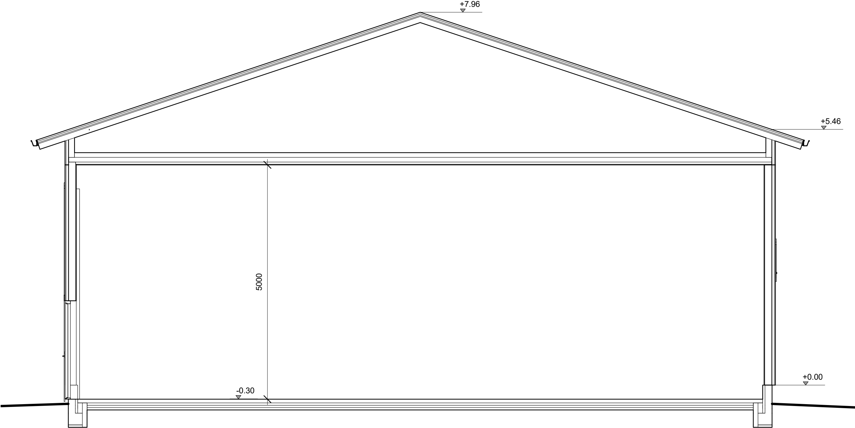
LEIKKAUS A-A
