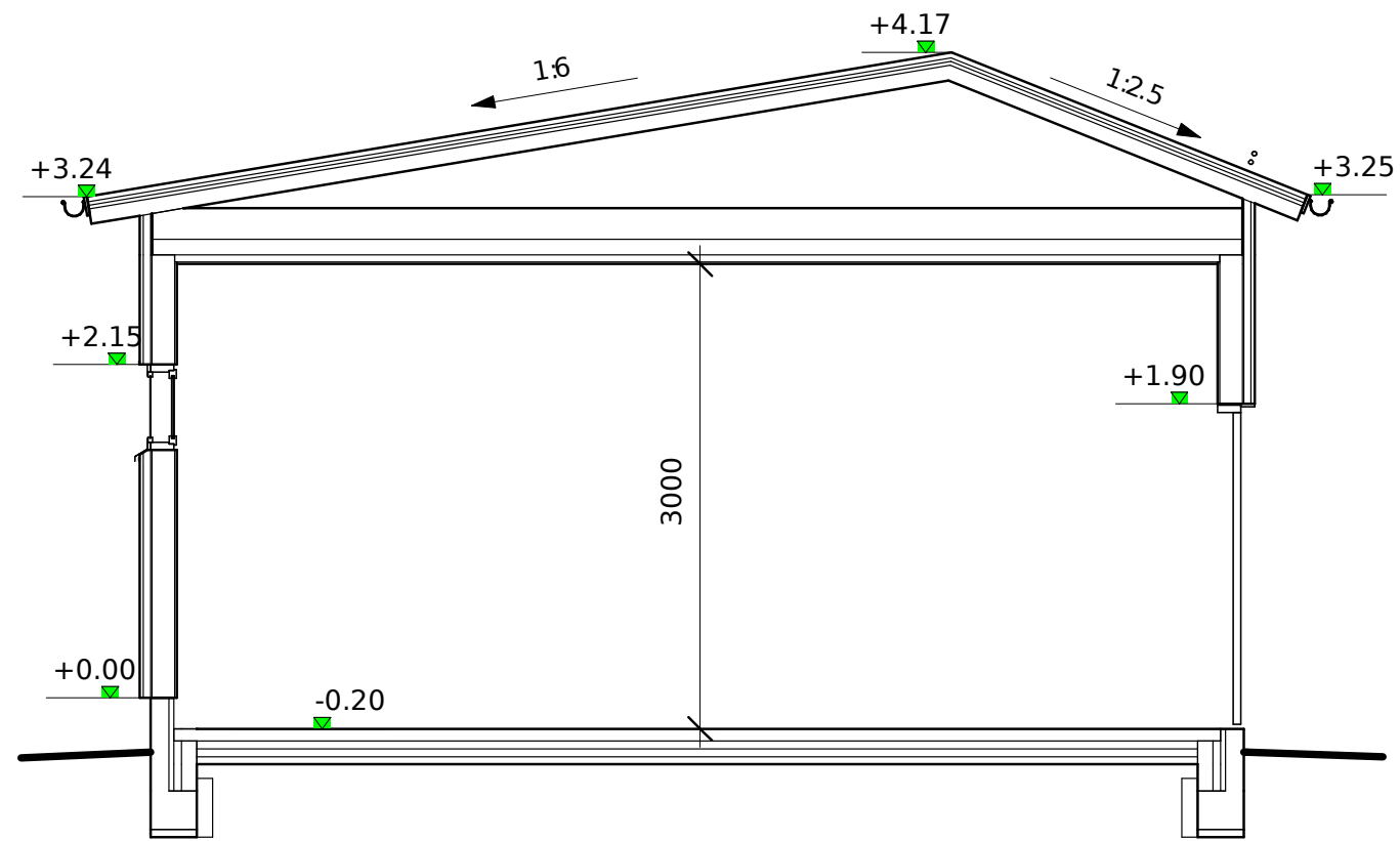
LEIKKAUS A-A
