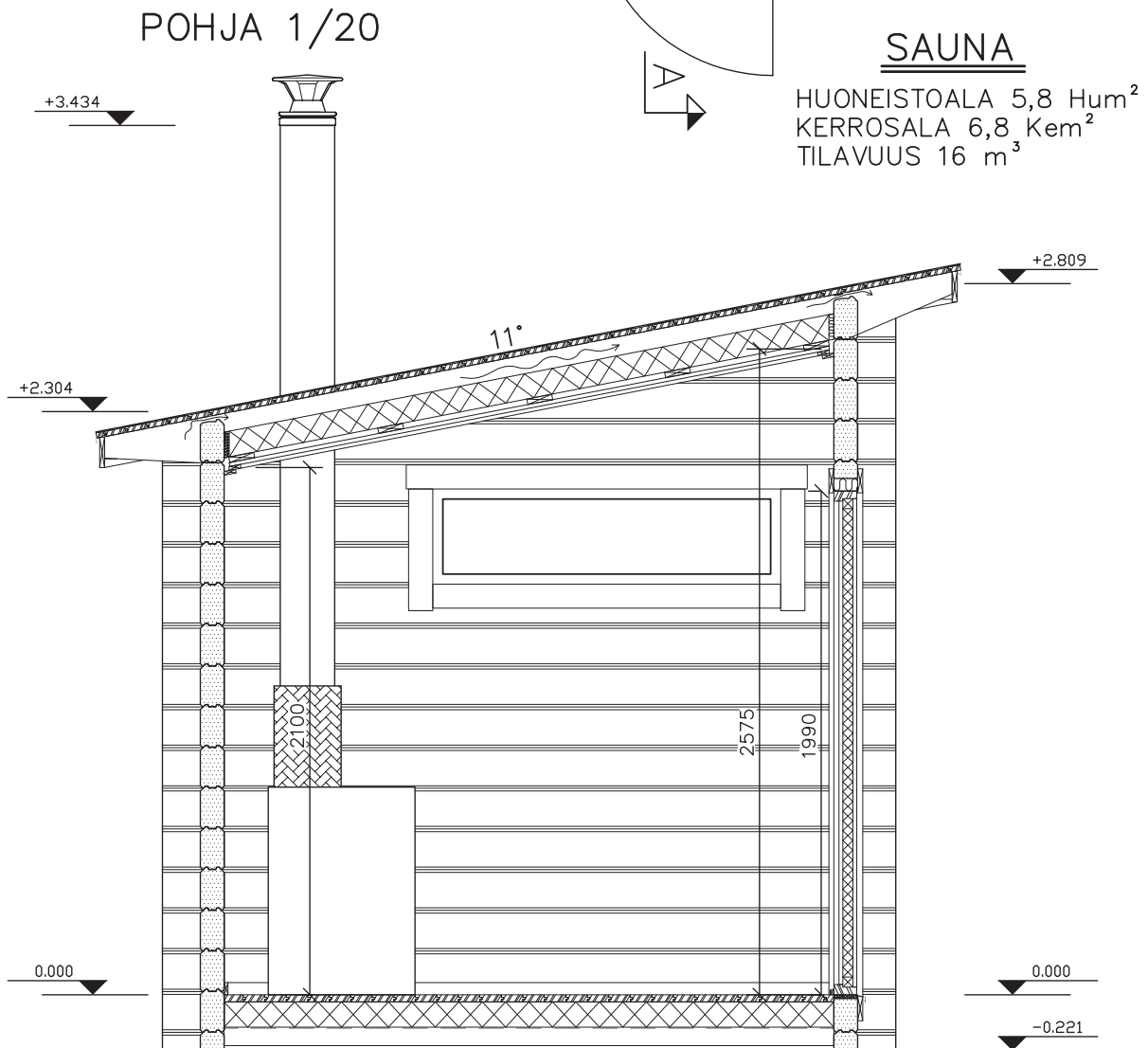
LEIKKAUS A-A
