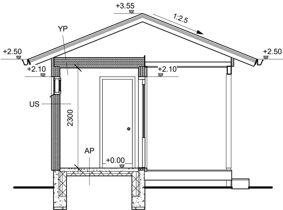
LEIKKAUS A-A
