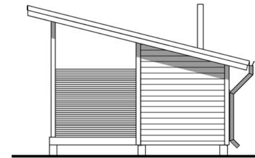
Julkisivu 3
