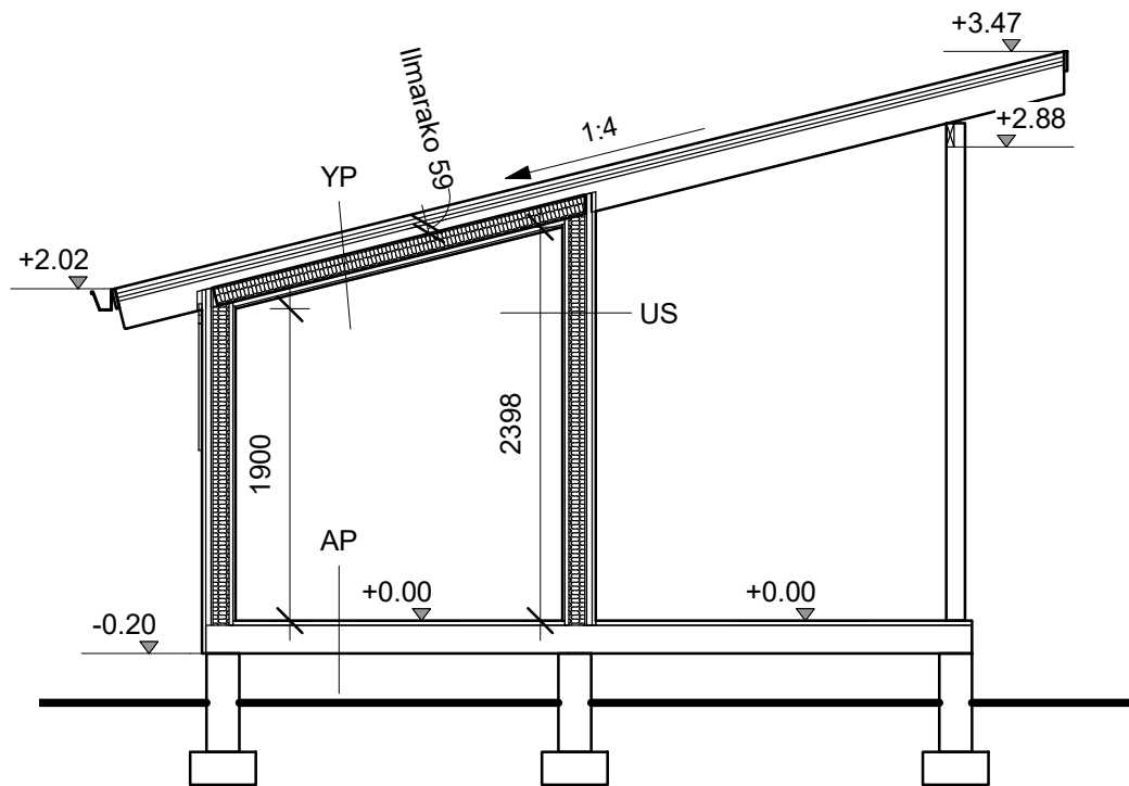
LEIKKAUS A-A
