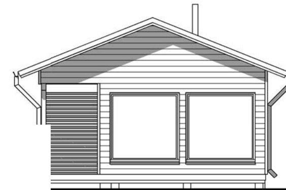
Julkisivu 3
