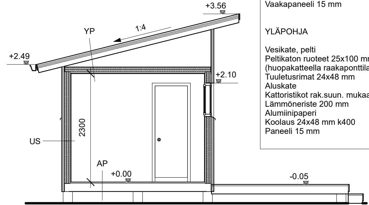
LEIKKAUS A-A
