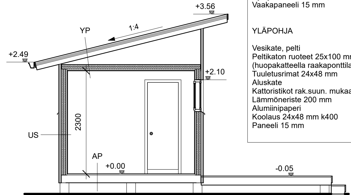
LEIKKAUS A-A
