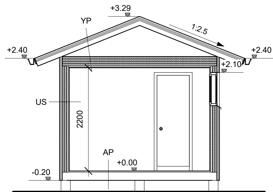
LEIKKAUS A-A
