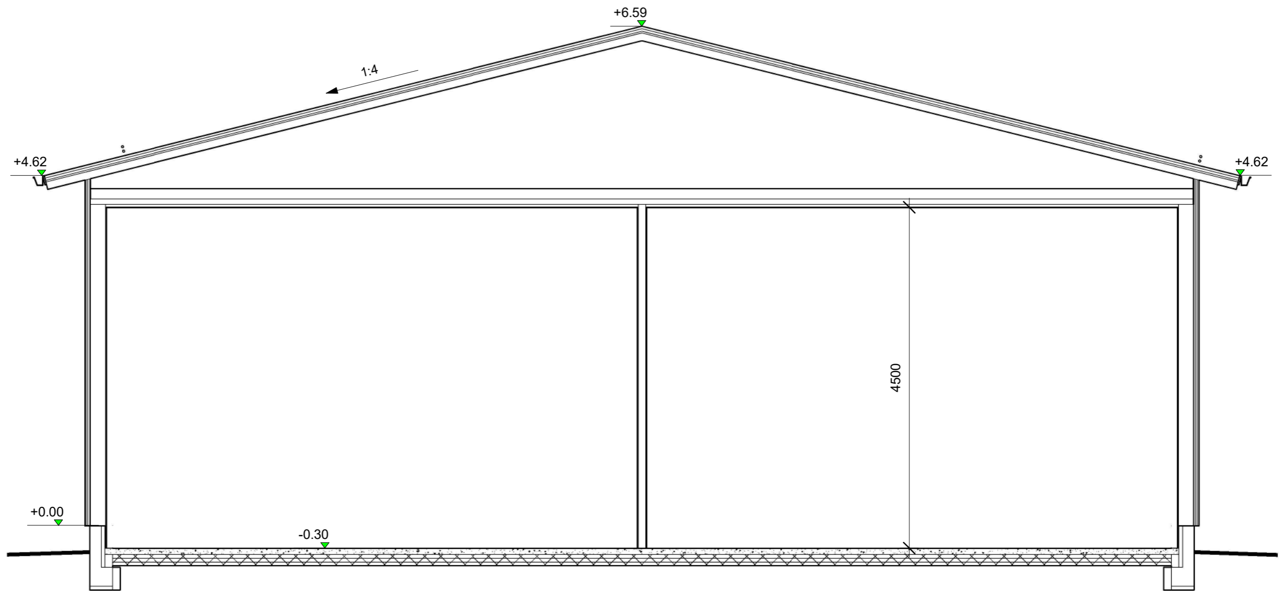
LEIKKAUS A-A
