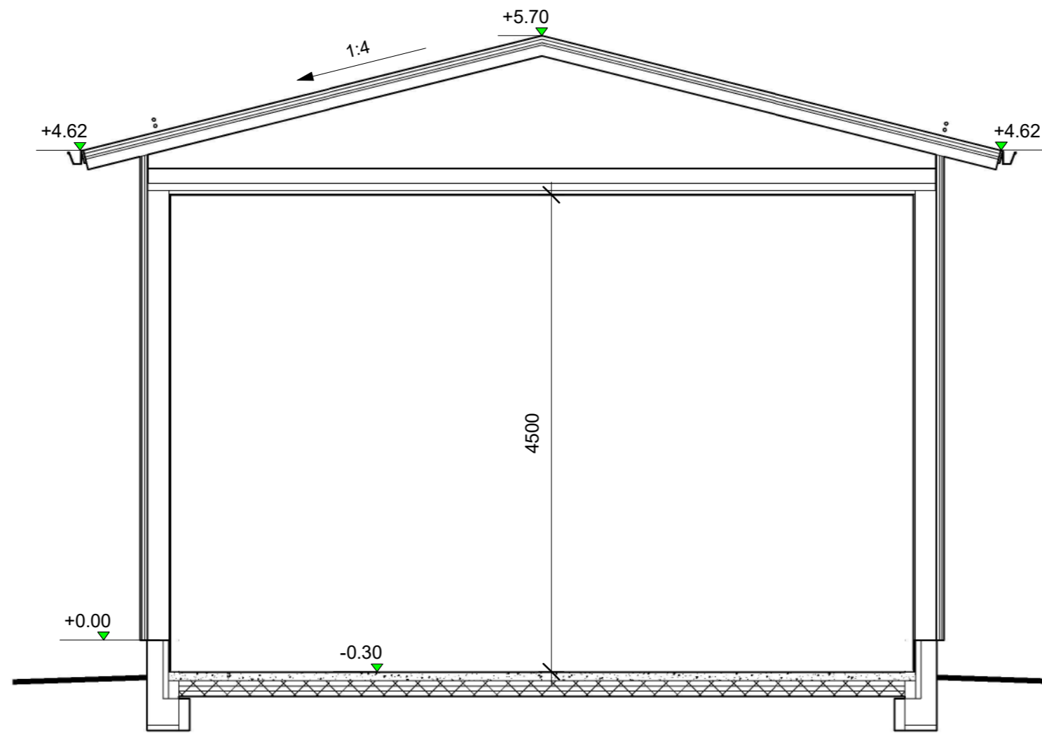
LEIKKAUS A-A
