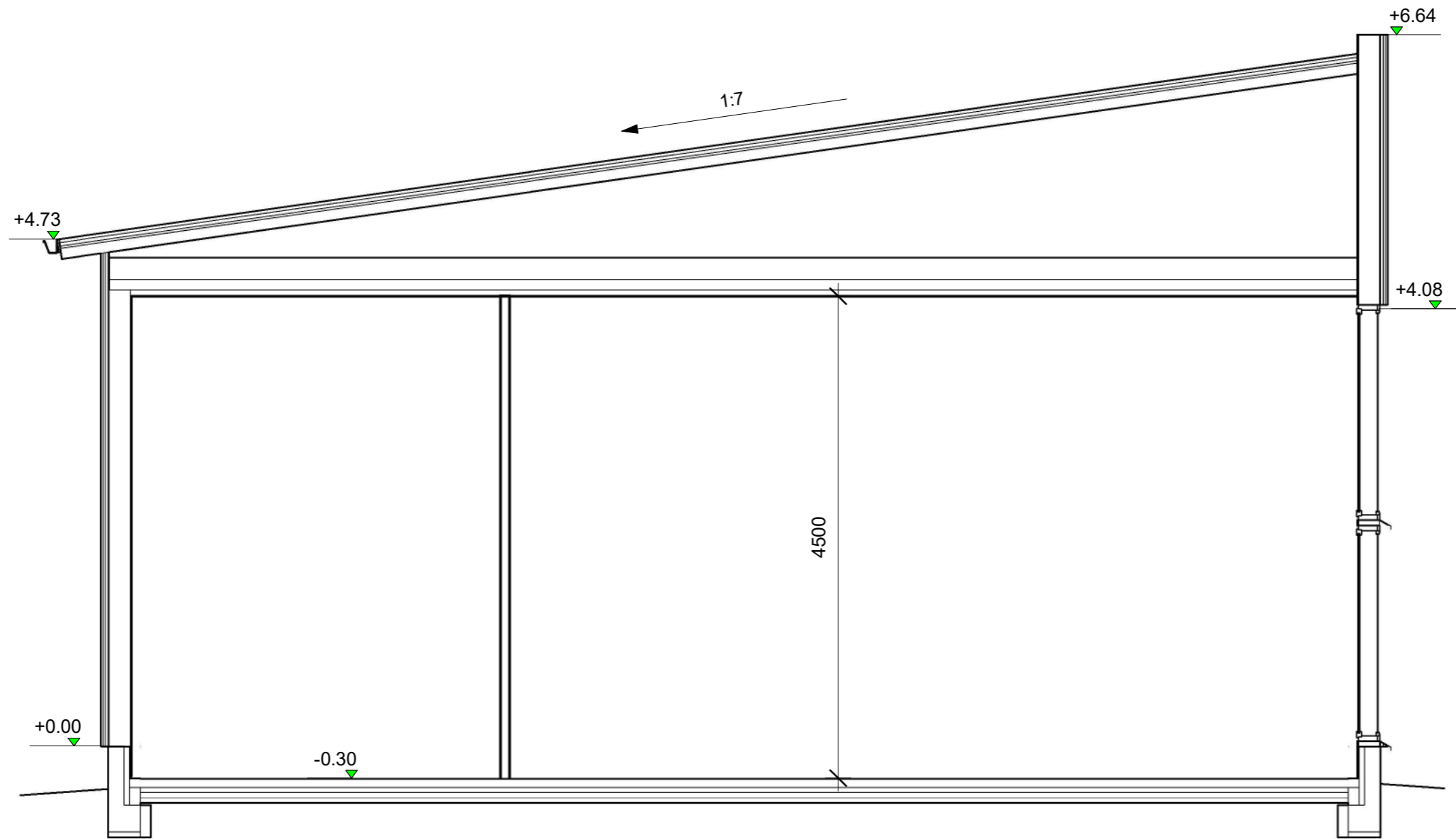
LEIKKAUS A-A
