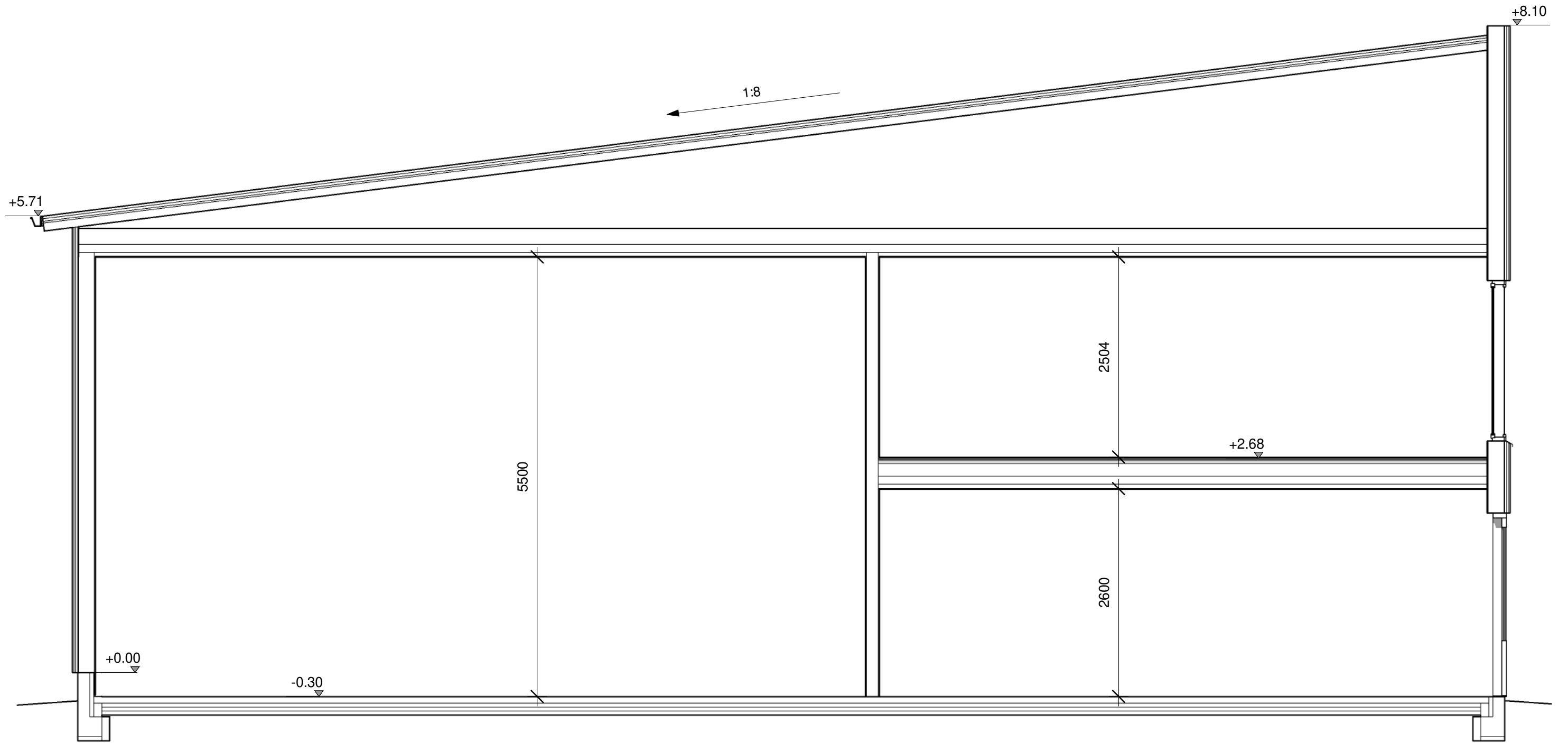
LEIKKAUS A-A
