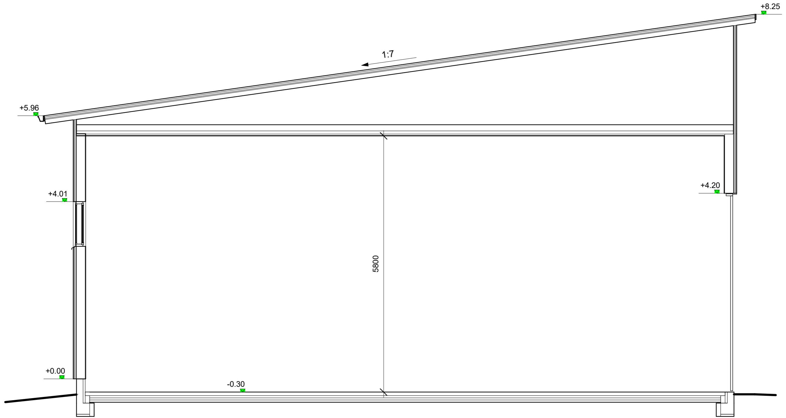
LEIKKAUS A-A
