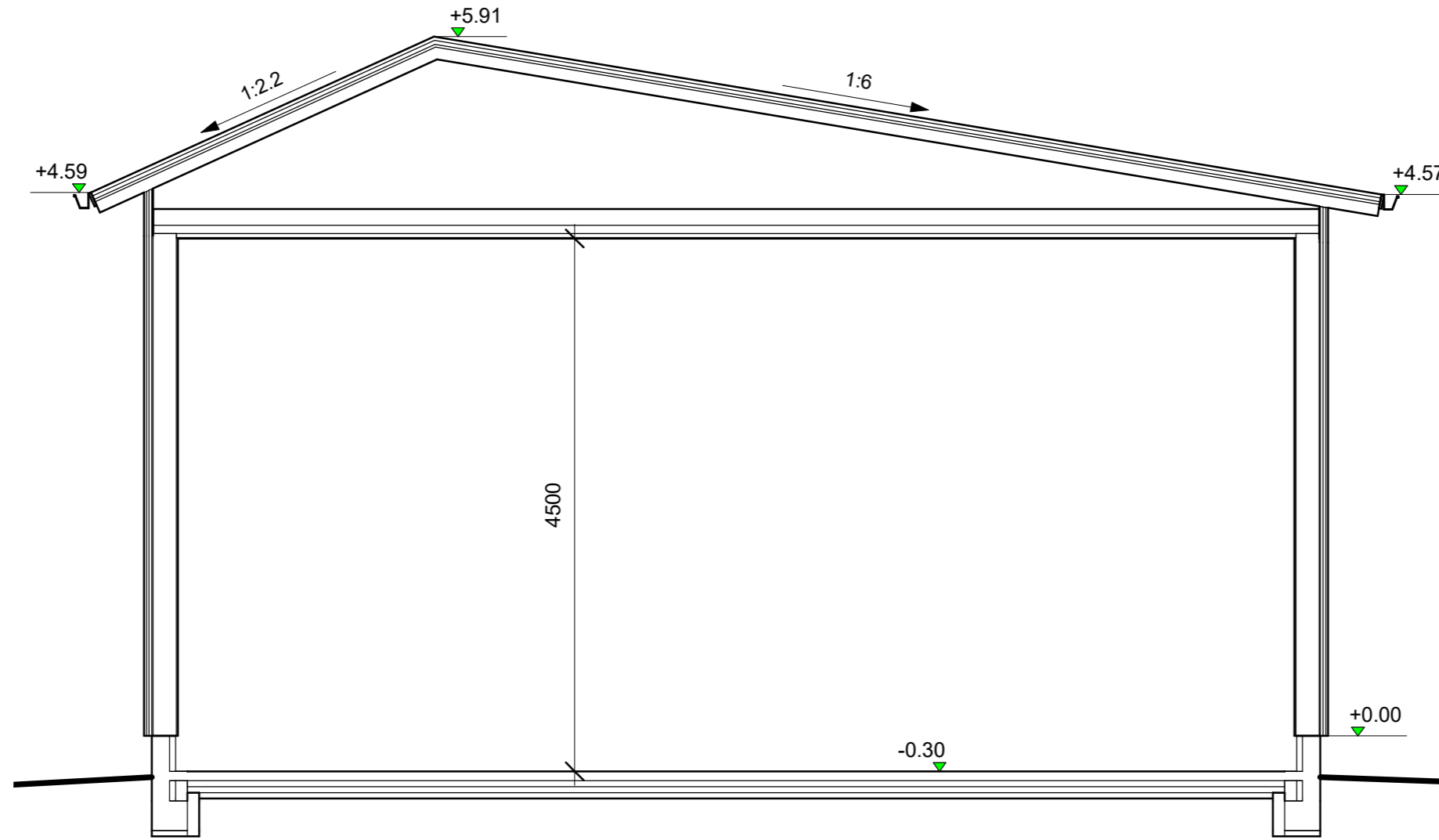
LEIKKAUS A-A
