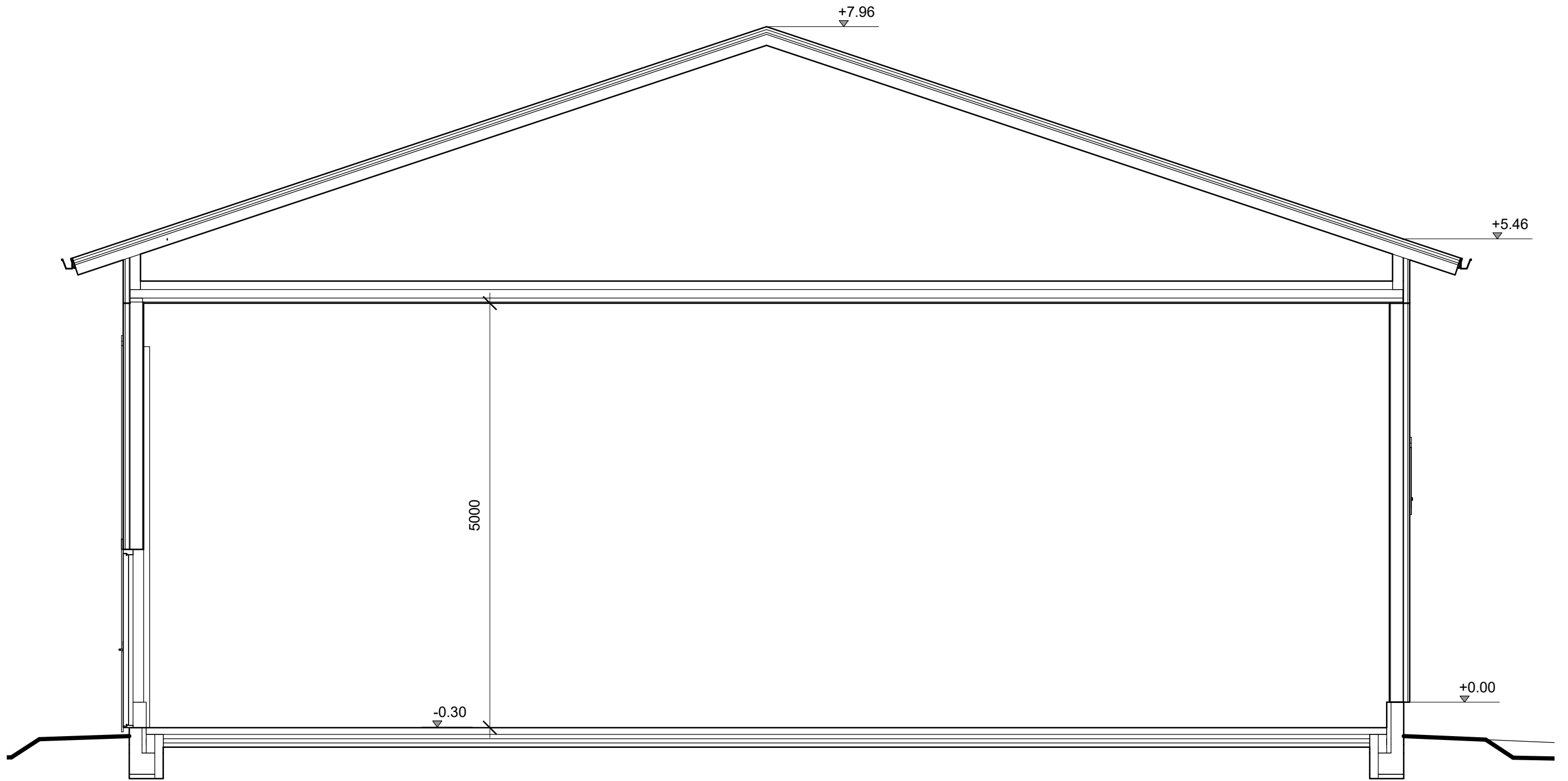
LEIKKAUS A-A
