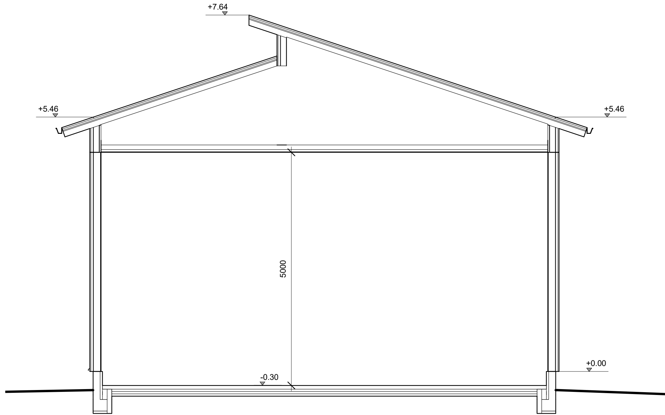
LEIKKAUS A-A
