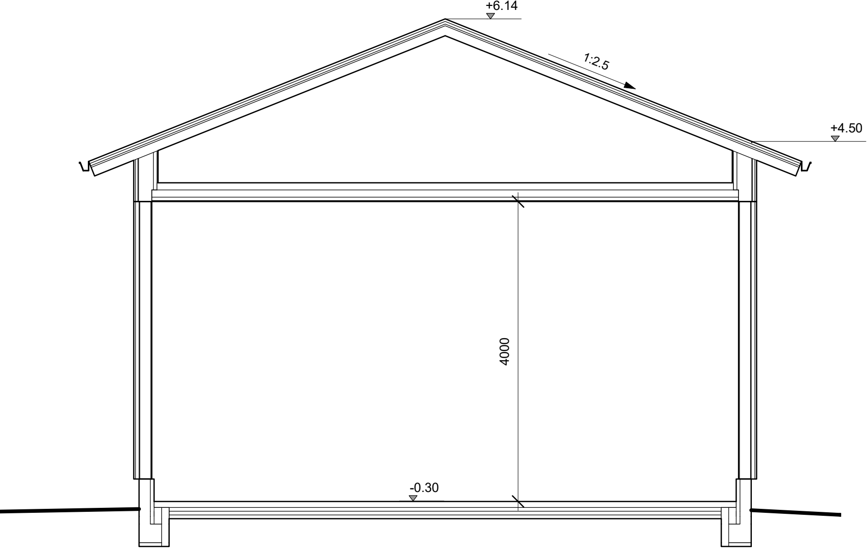
LEIKKAUS A-A
