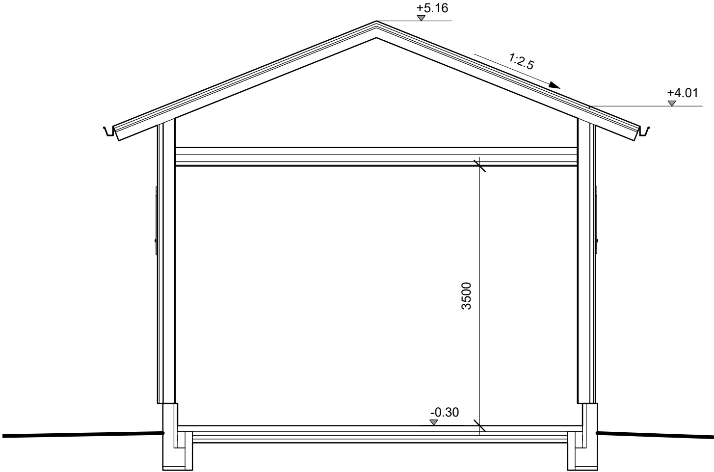
LEIKKAUS A-A
