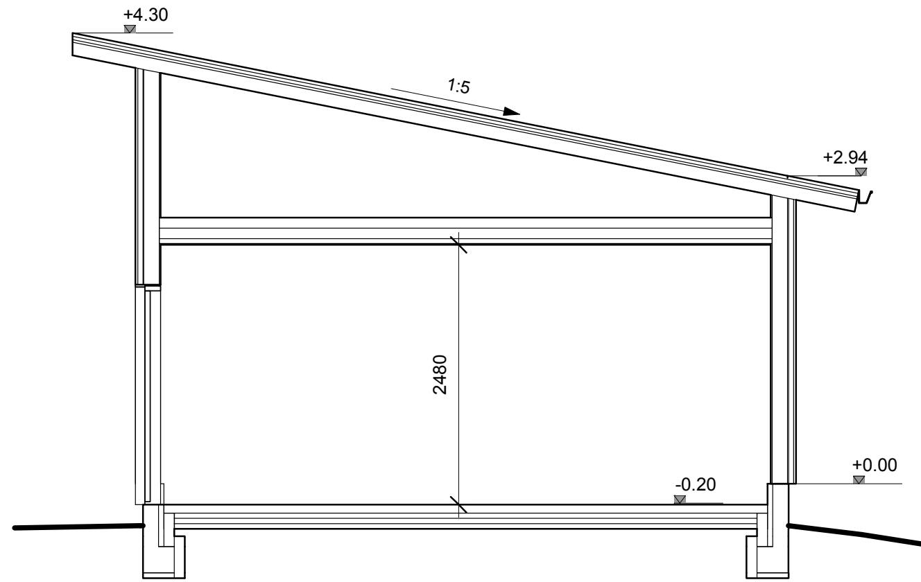
LEIKKAUS A-A
