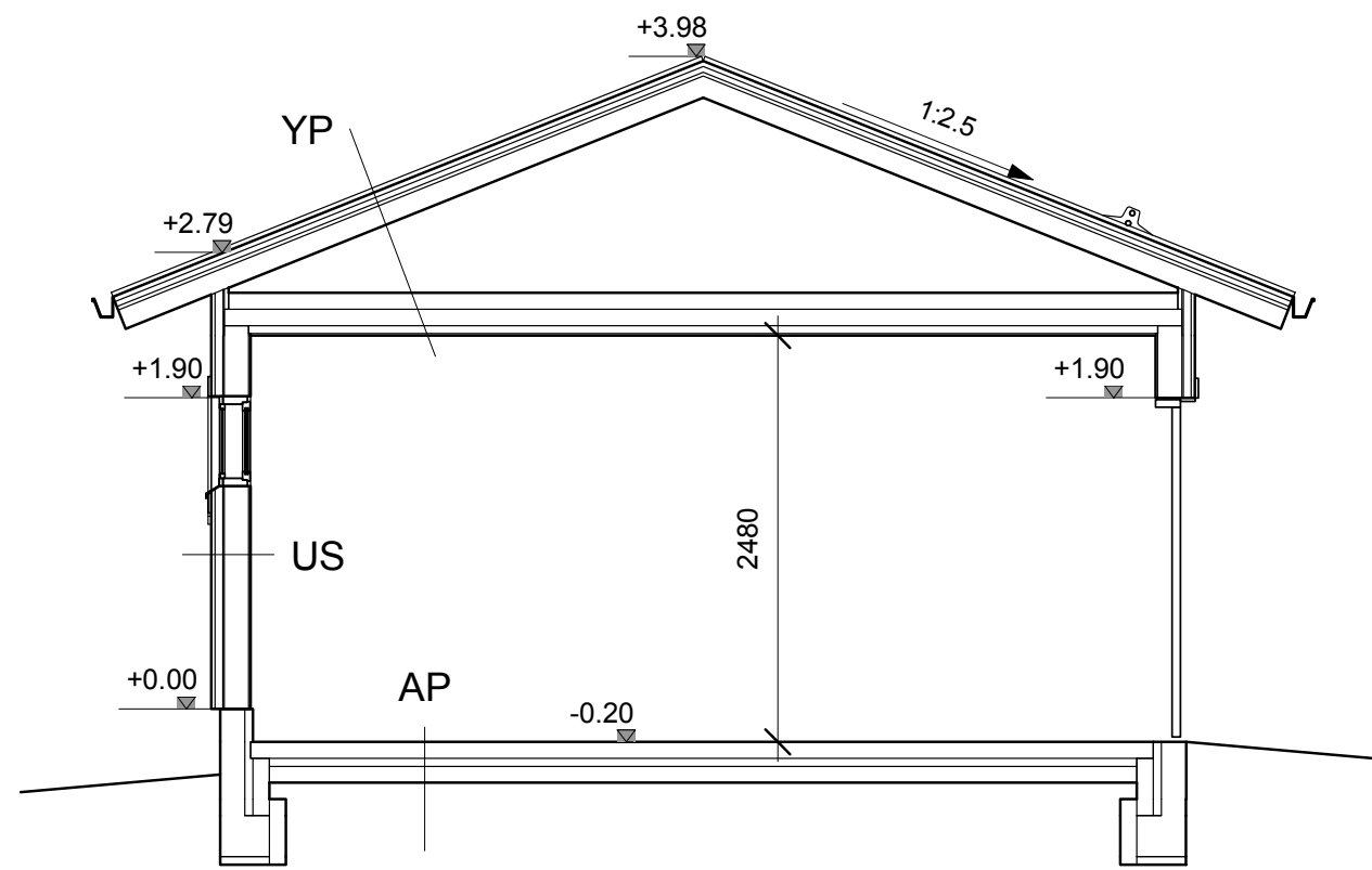
LEIKKAUS A-A
